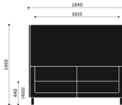
VL3 HW / VL3 VW + VL W3
