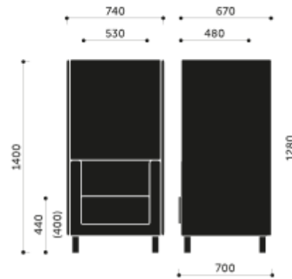
VL1 HW / VL1 VW + VL W1
