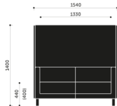
VL2,5 HW / VL2,5 VW + VL W2,5
